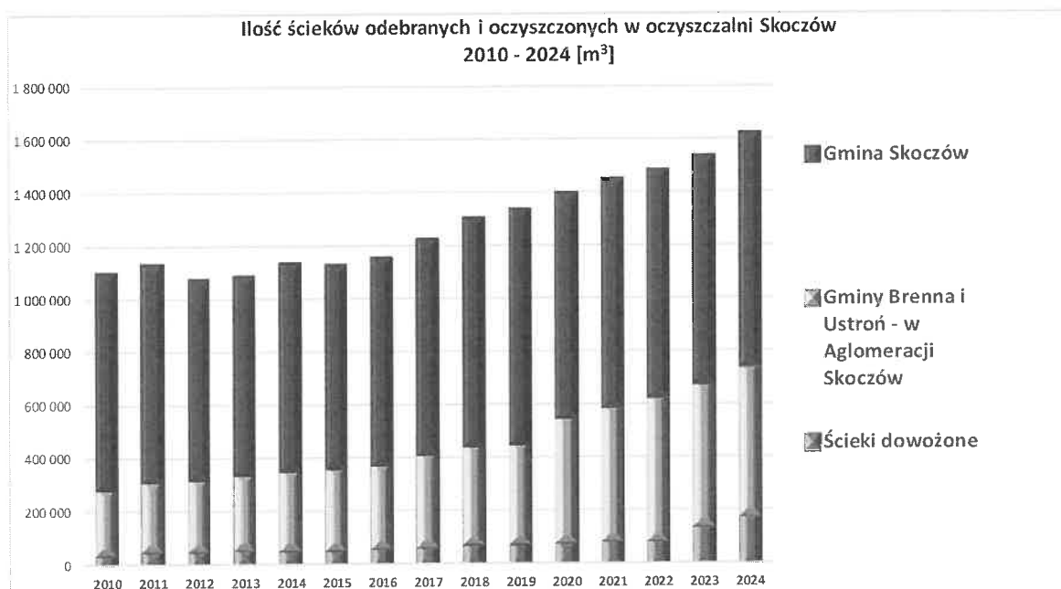
Graficzna prezentacja odbioru i oczyszczania ścieków w oczyszczalni Skoczów
